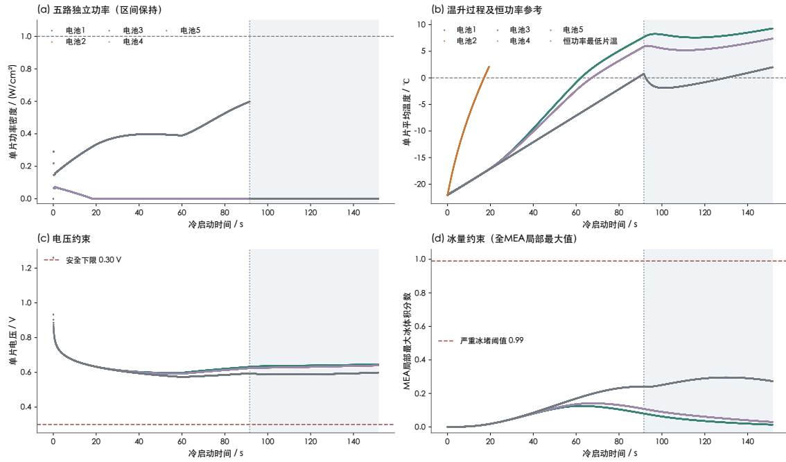
工况3：预冷40 min | 推荐动态全过程；阴影为关热后验证 功率圆点对应前一积分区间的实际加热；所有时刻均保留，圆点之间不连线。
