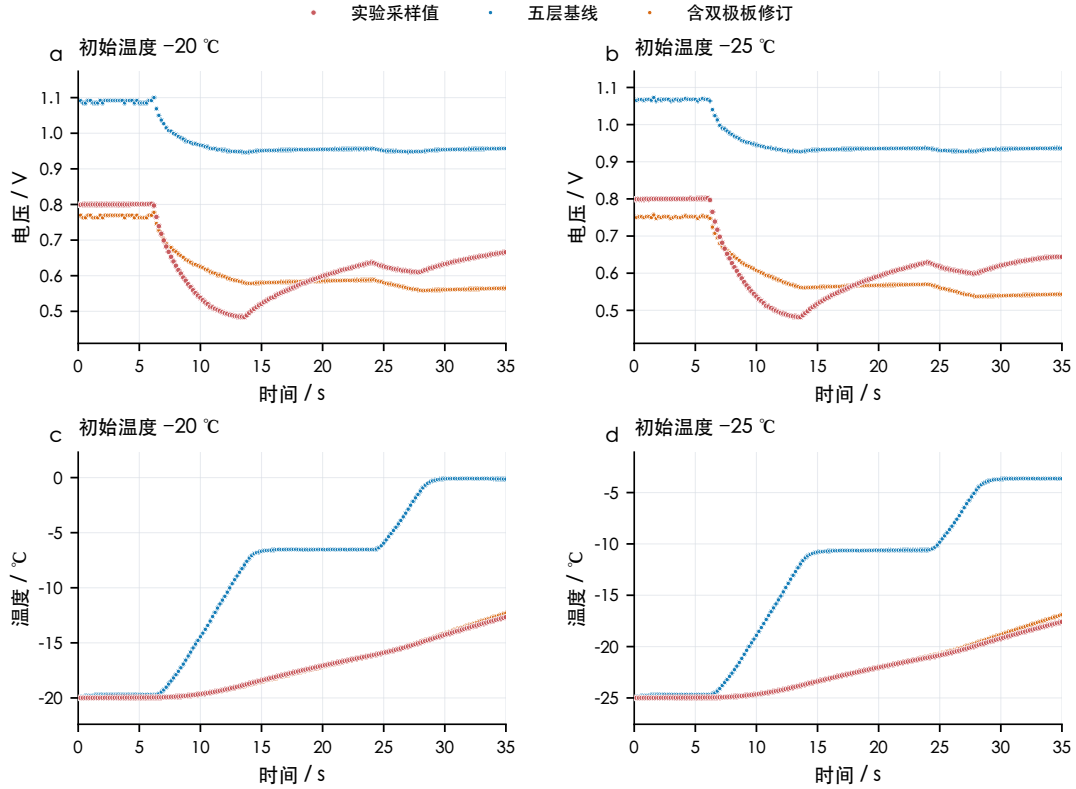
图 4-2 实验数据与五层基线与含双极板修订模型对比图
