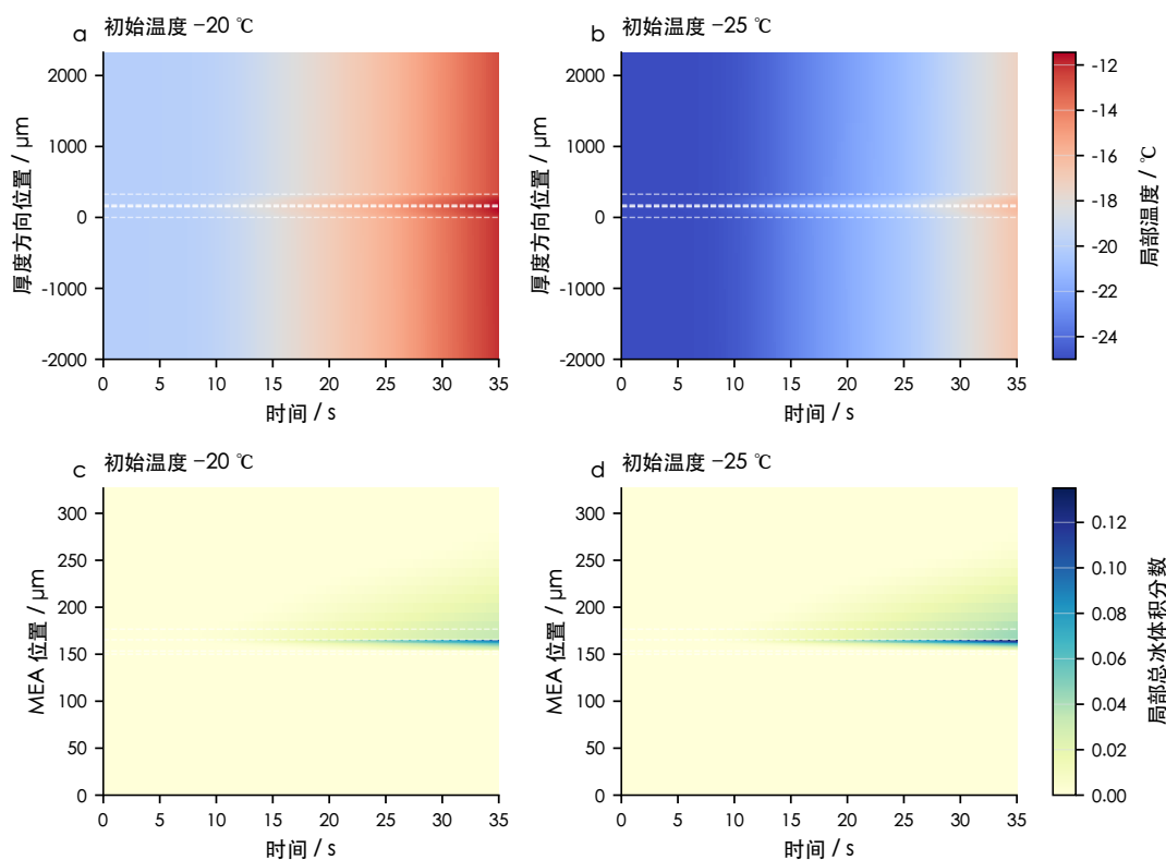
图 4-4 含双极板修订模型温度与结冰时空分布图
