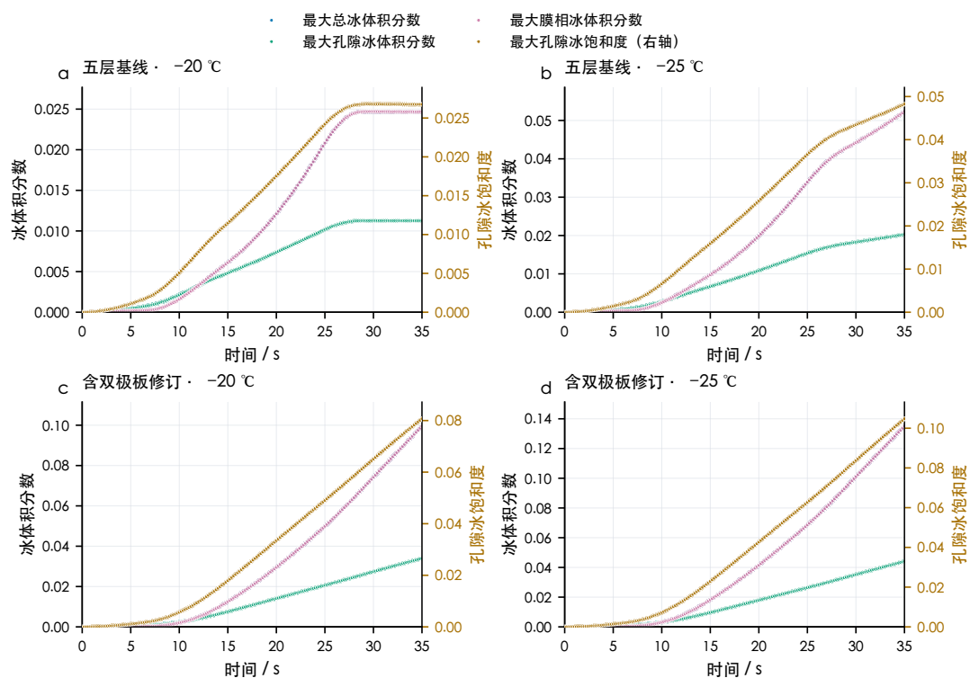
图 4-3 总冰孔隙冰膜相冰体积分数与孔隙冰饱和度图
