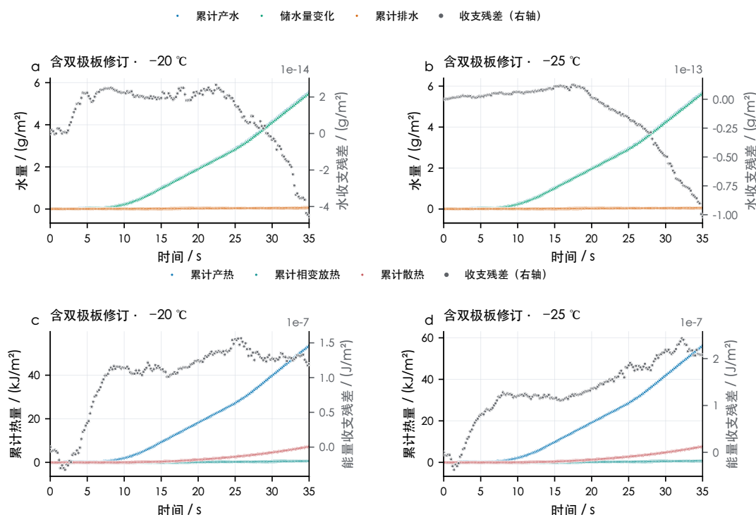
图 4-5 含双极板模型水量热量收支与守恒残差图
