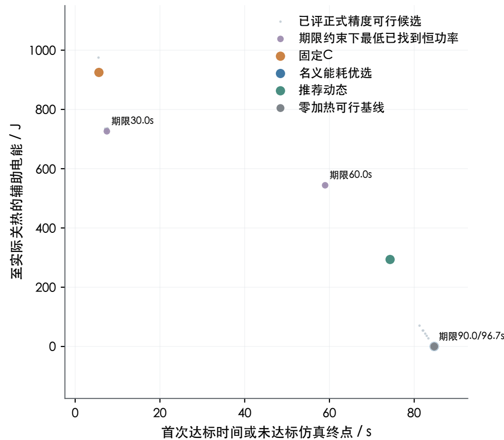
(b) 工况2：预冷20 min
