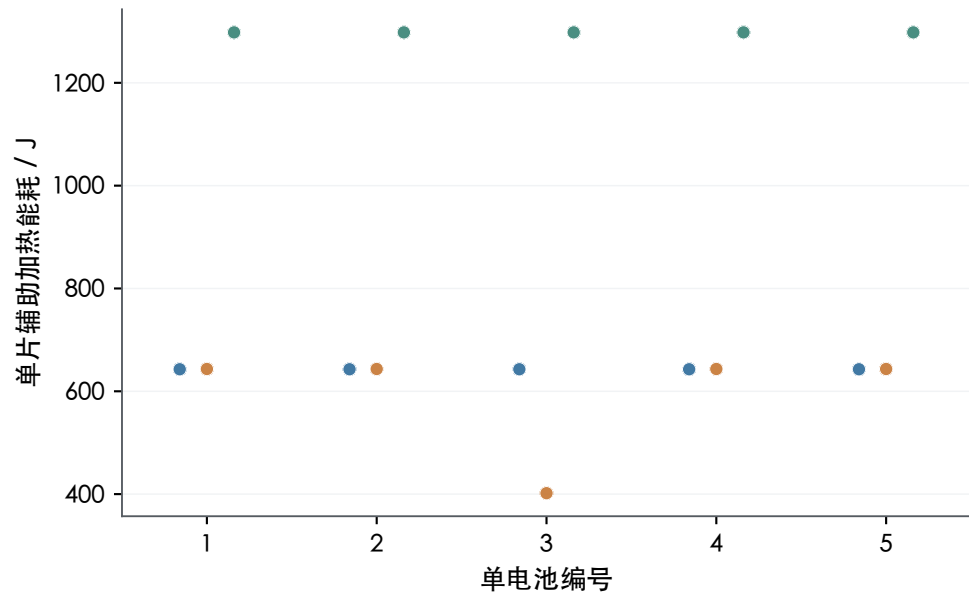
(b) 各片累计辅助能耗
