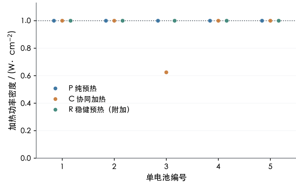
(a) 各片恒定加热功率
