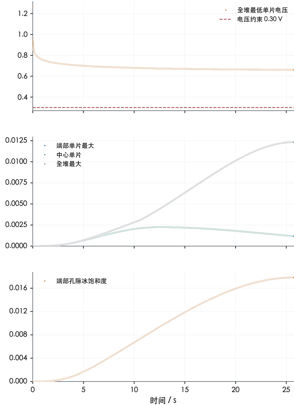
(b) C 协同加热
