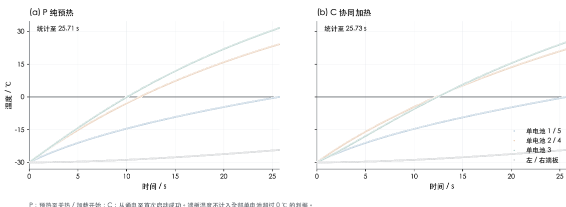
图 6-2 两种主策略温度历程图
