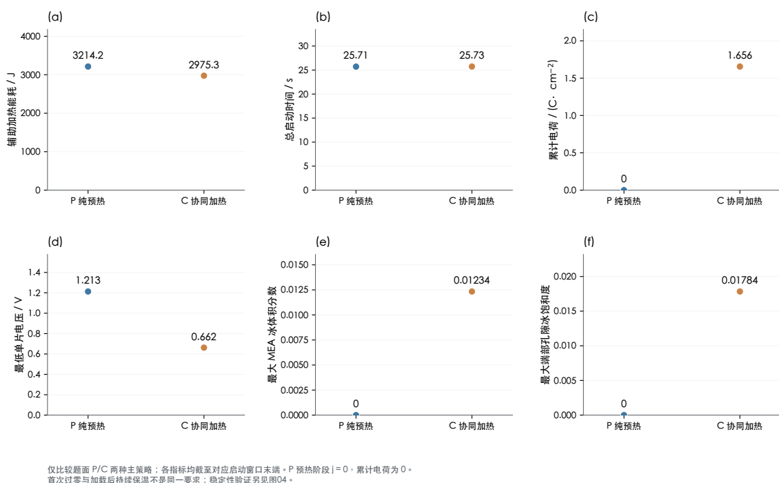
图 6-1 两种主策略关键指标对比图
