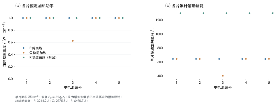
图 6-3 各片加热功率与辅助能耗分配图
