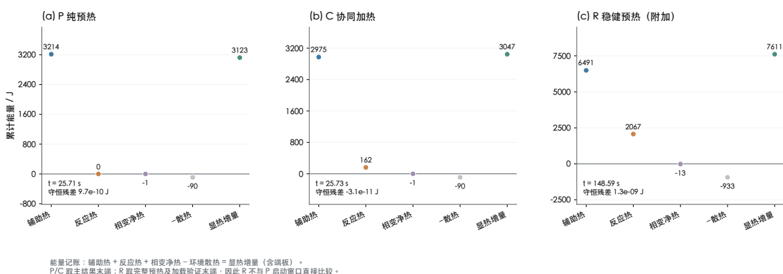
图 6-6 辅助冷启动能量预算与守恒检验图
