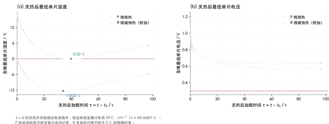
图 6-5 关热后温度回落与稳健预热验证图
