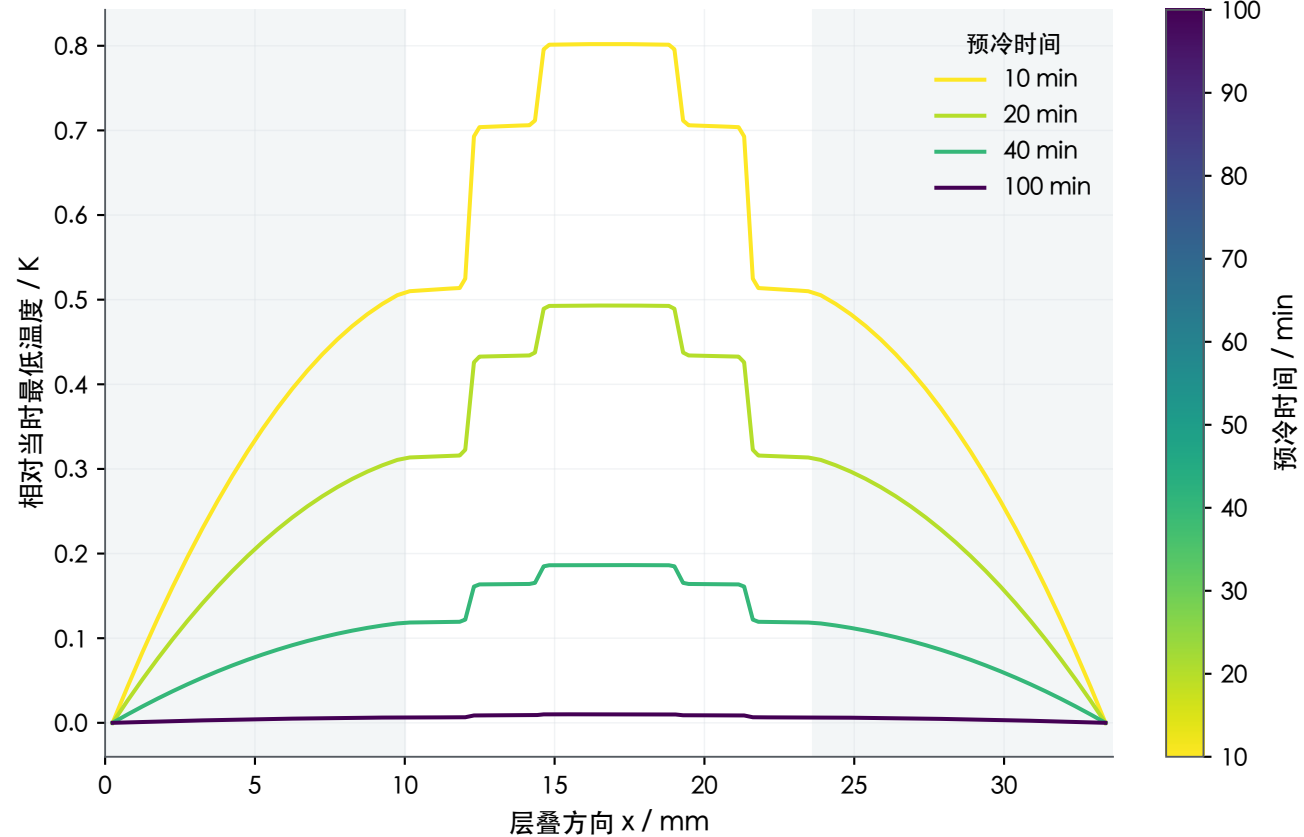
(b) 空间温差细节
