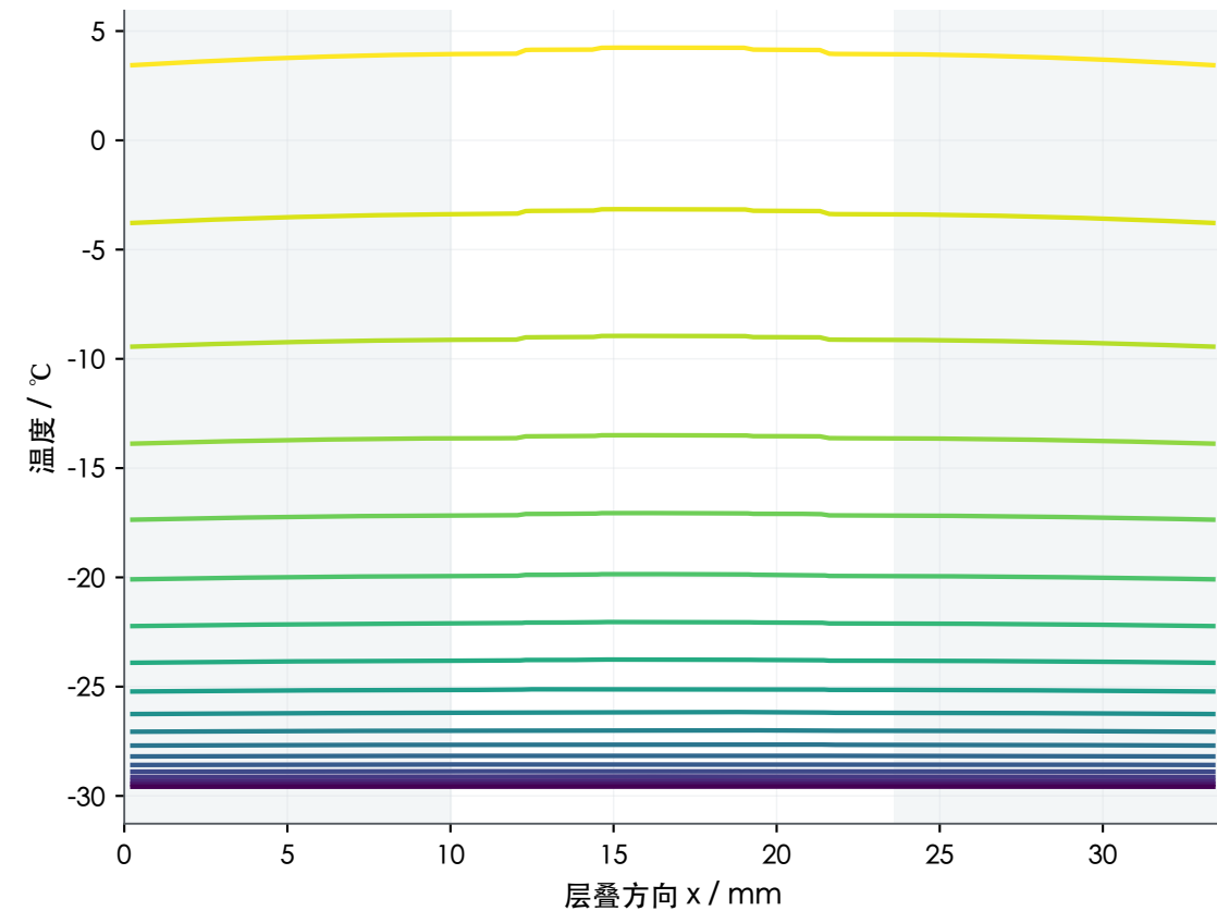
(a) 10-100 min 温度场族 (间隔5 min)
