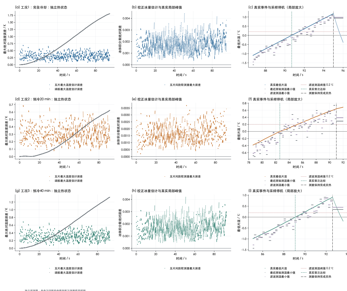
图 7-9 参数失配与测量噪声下的观测误差及停机事件辨析
