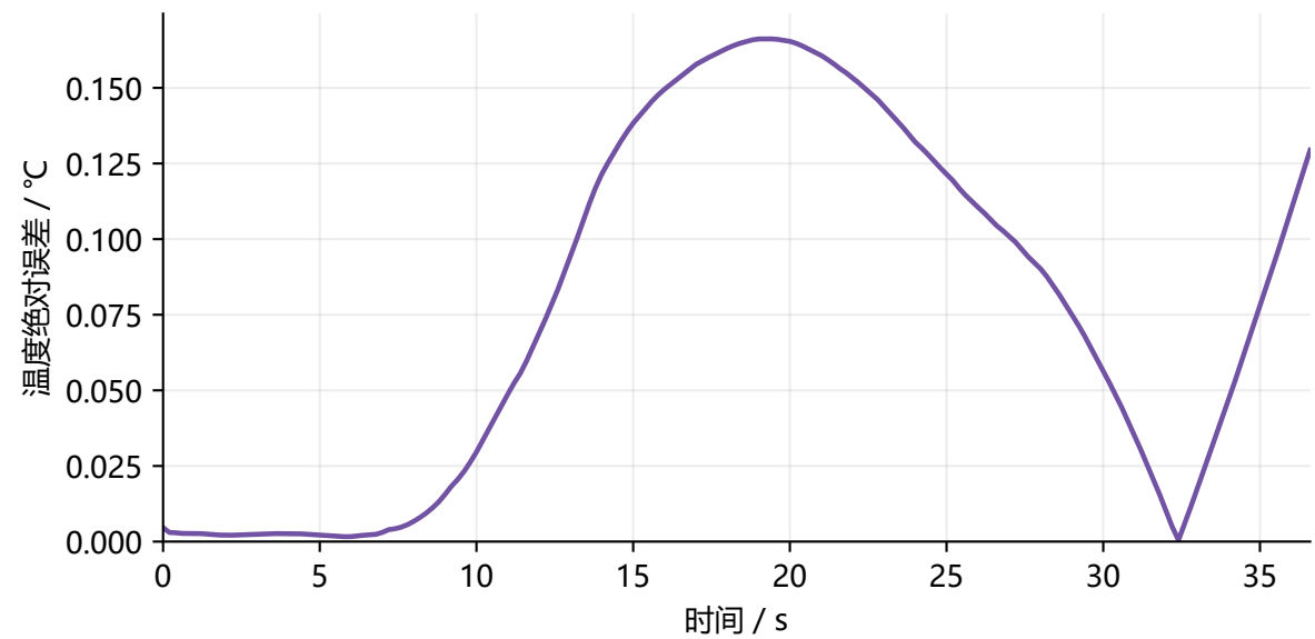
有效时段内的模型与实验绝对误差
