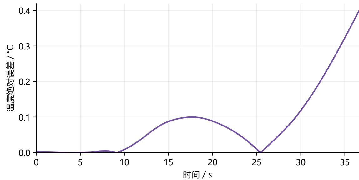
有效时段内的模型与实验绝对误差
