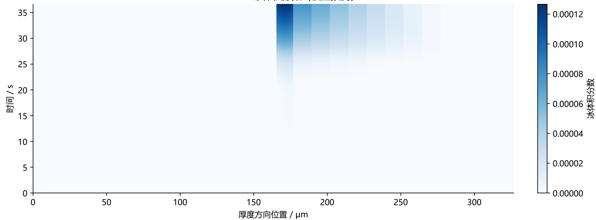
-25 °C — MEA冰体积分数 (模型预测)
