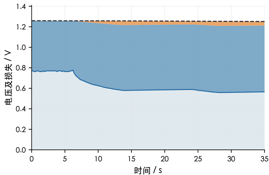
(c) 含双极板修订 · -20 °C
