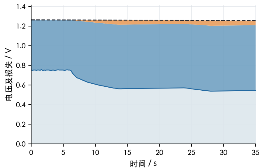
(d) 含双极板修订 · -25 °C
