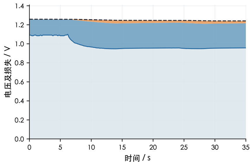
(a) 五层基线 · -20 °C
