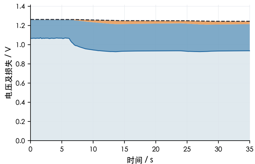
(b) 五层基线 · -25 °C
