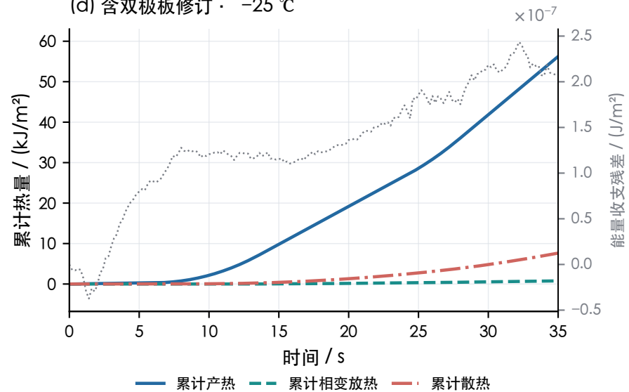
(d) 含双极板修订 · -25^{\circ}\text{C}
