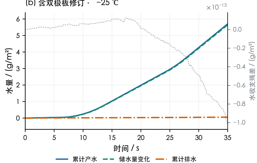
(b) 含双极板修订 · -25^{\circ}\text{C}
