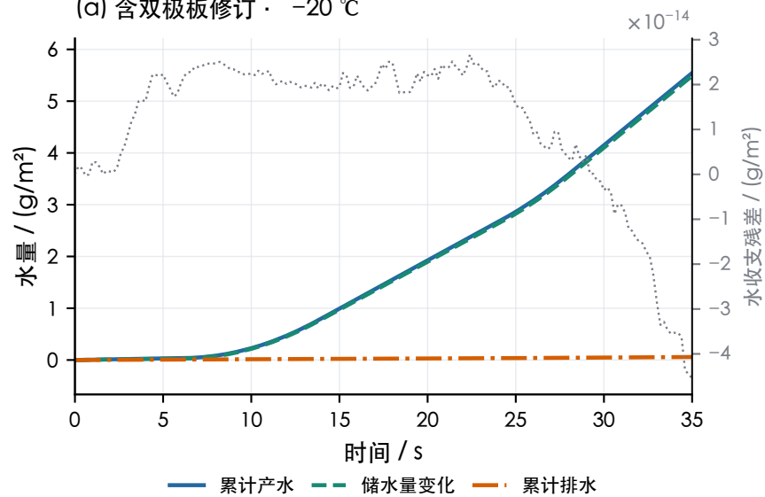
(a) 含双极板修订 · -20^{\circ}\text{C}
