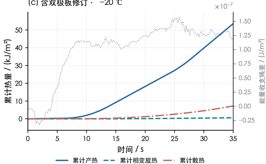
(c) 含双极板修订 · -20^{\circ}\text{C}
