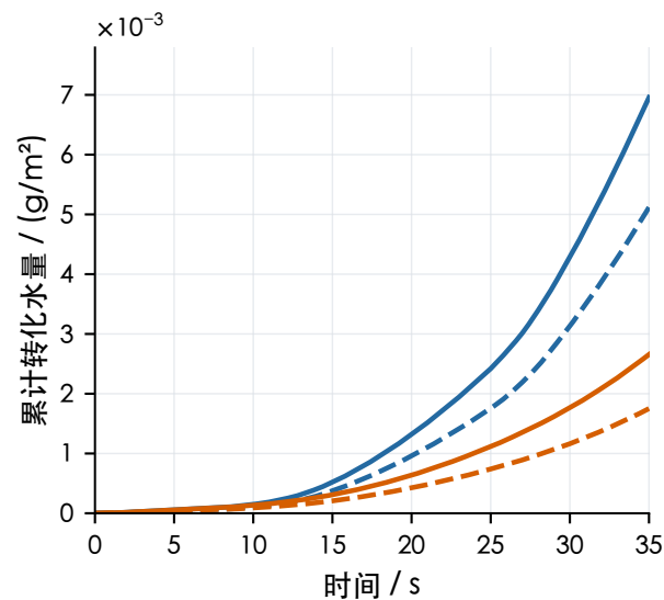
(b) 蒸发
