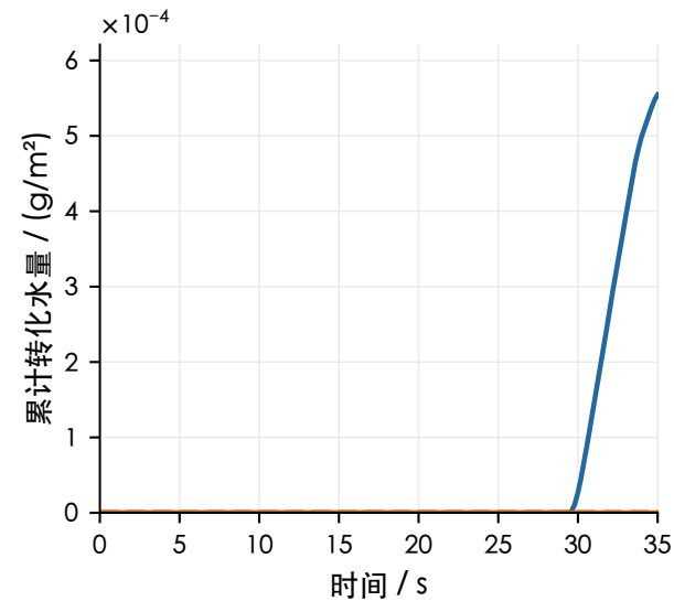
(f) 融化
