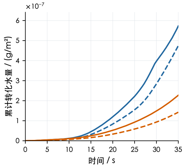
(d) 升华
