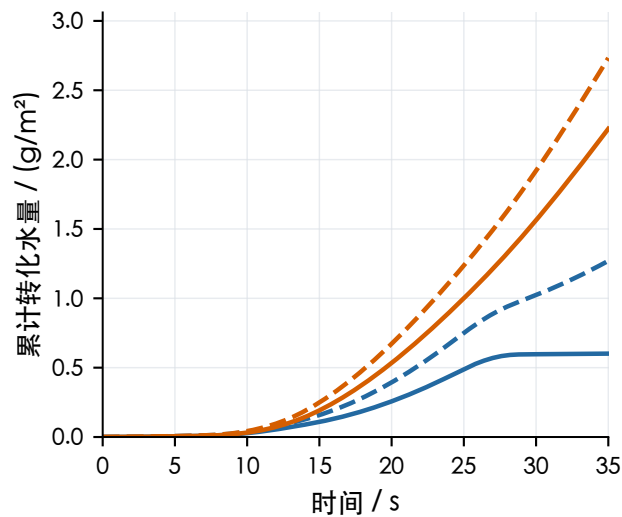
(e) 冻结
