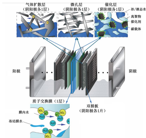
图 1 氢燃料电池冷启动时主要传输现象示意图 [2]
