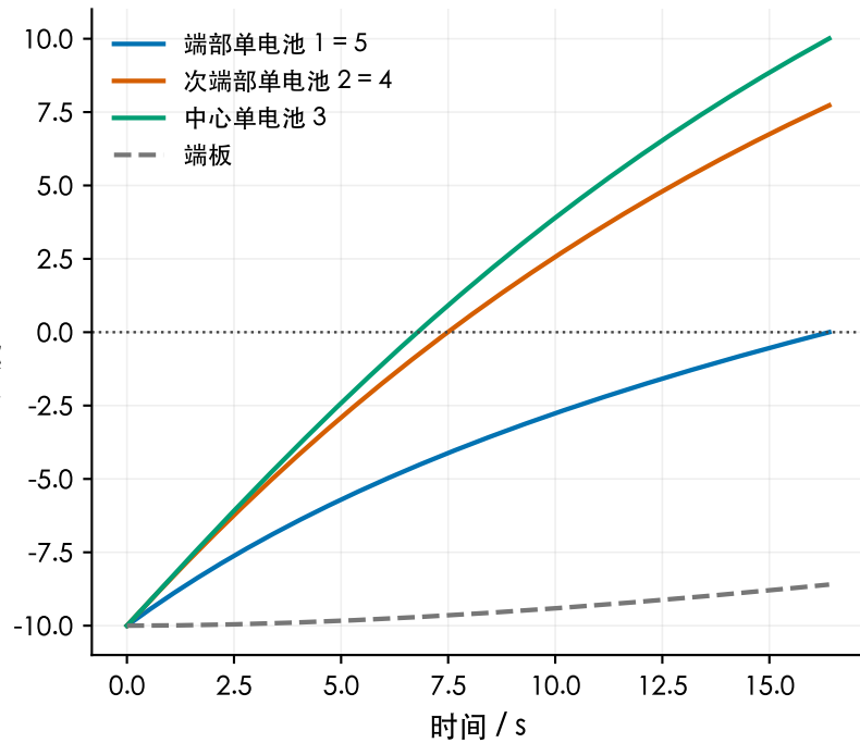
恒流加载
