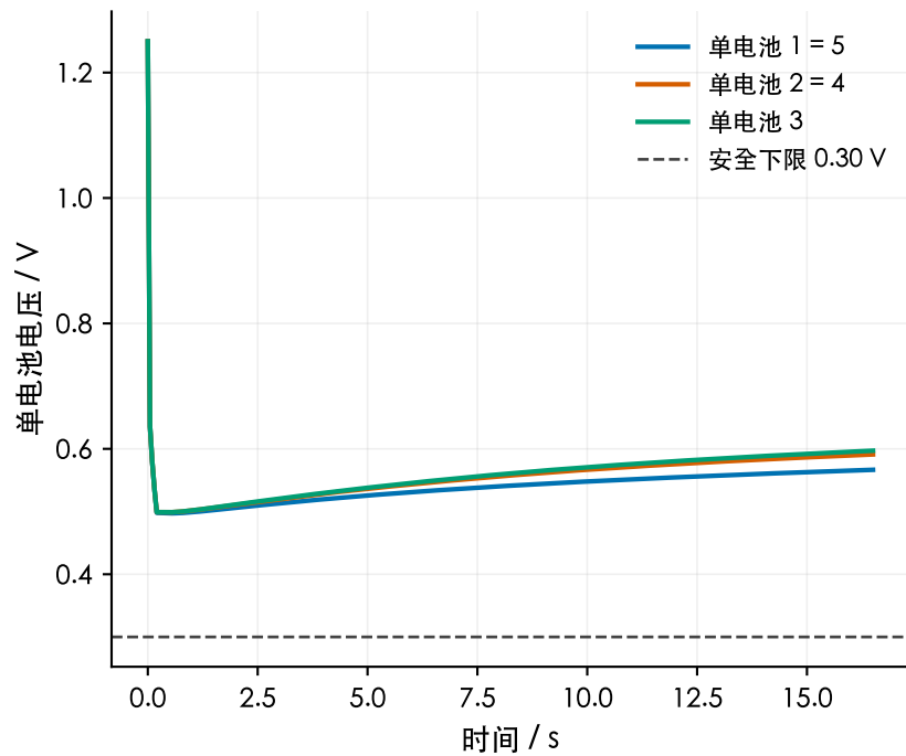
线性斜坡加载
