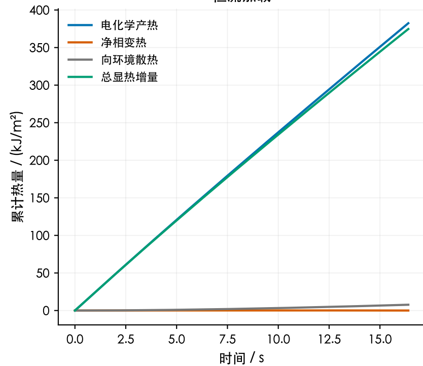
恒流加载
