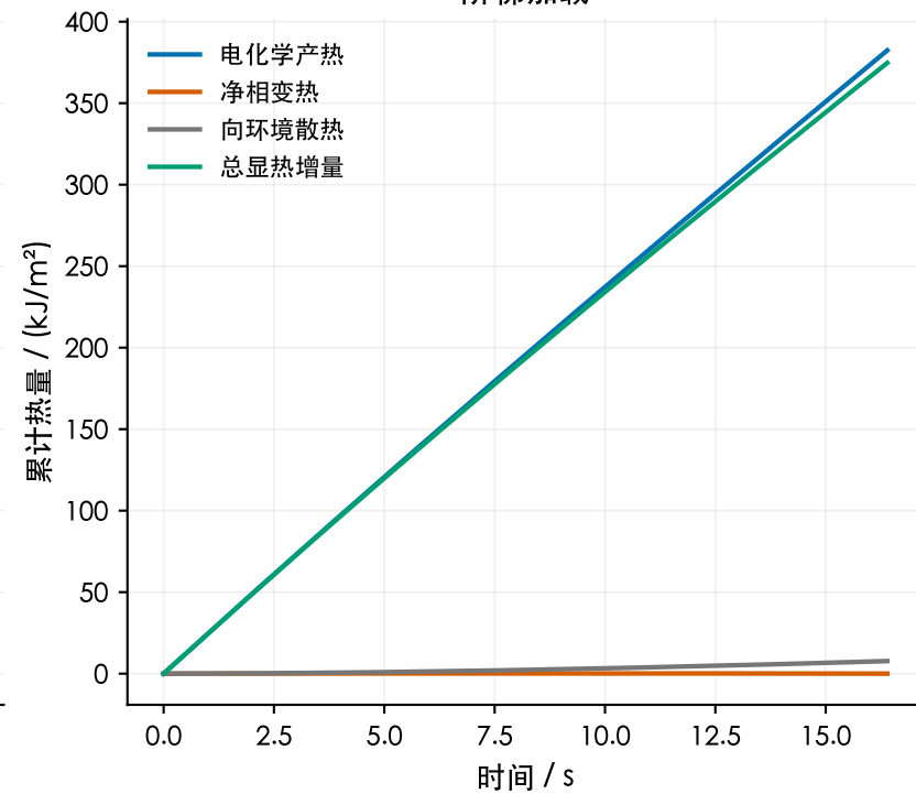
阶梯加载
