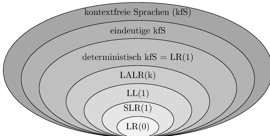
Abbildung 4.8.: Sprachenhierarchie
