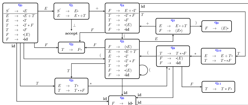
Abbildung 4.5.: Parser-Automat
