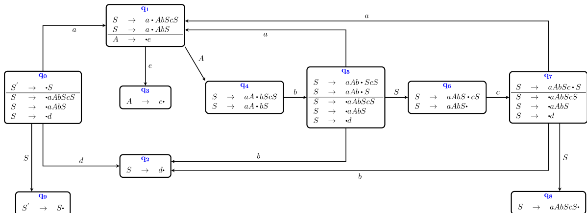
Abbildung 4.6.: LR(0)-Automat
