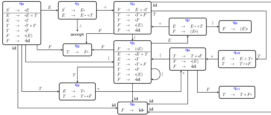
Abbildung 1: Parser-Automat
