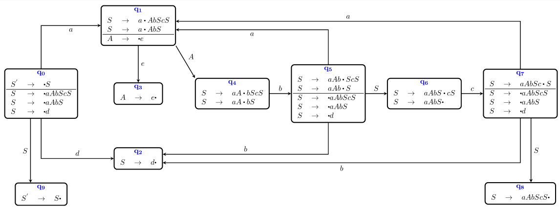
Abbildung 2: LR(0)-Automat
