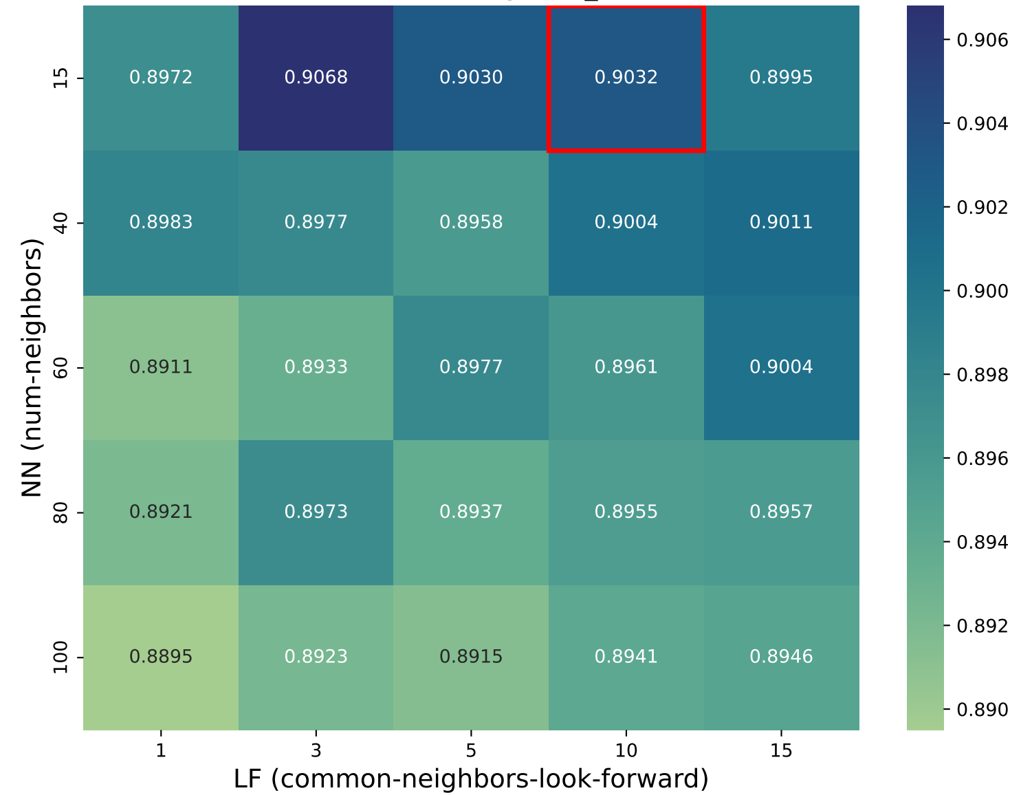
WikiRfA · linksign · f1_wt
