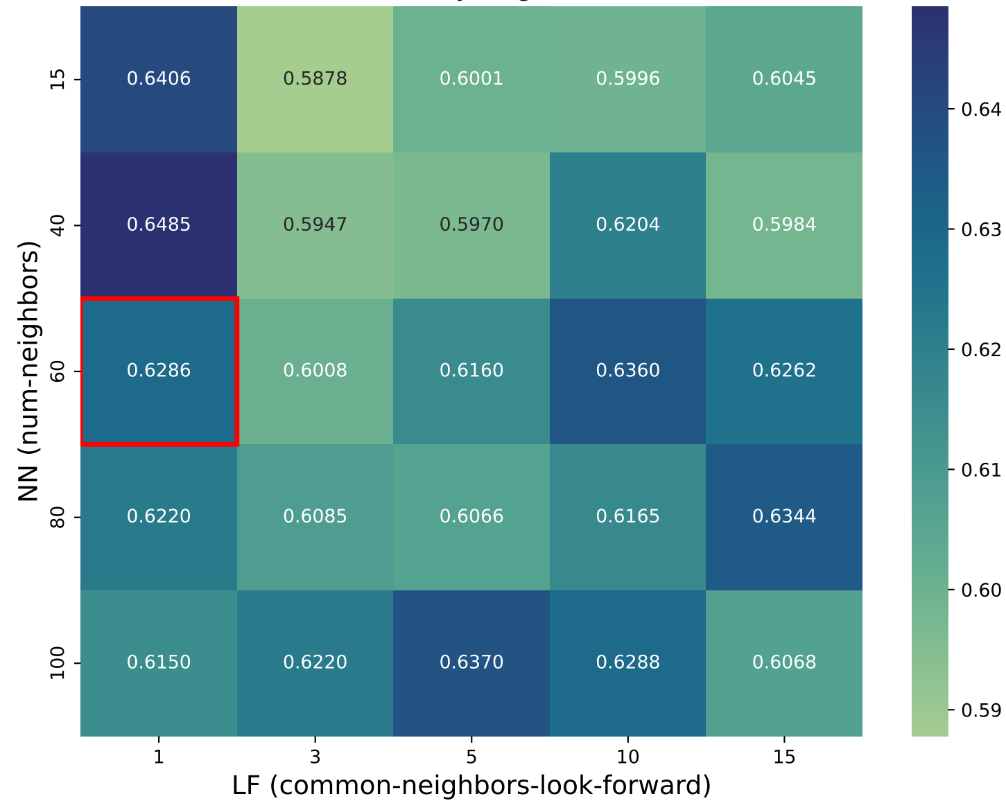
RedditBody · sign · auc
