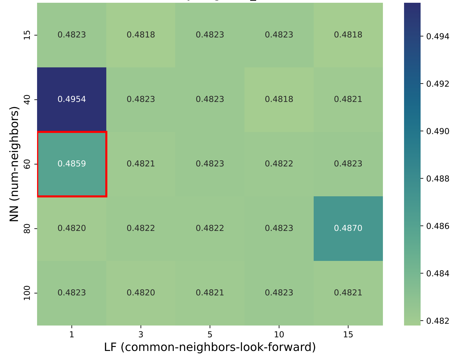
RedditBody · sign · f1_macro
