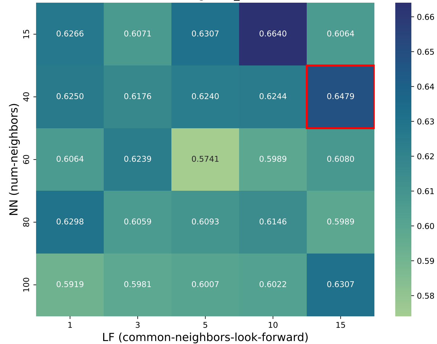
WikiRfA · sign · f1_macro
