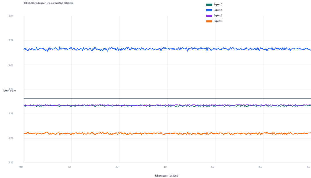
Figure 7: Utilisation des experts pendant le run Token-Routed 300M corrigé. Les quatre experts restent actifs et proches de l’équilibre ; le gain observé ne vient pas d’un effondrement d’expert.
