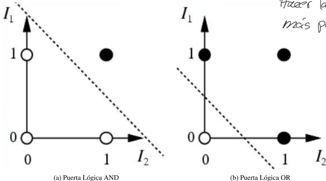
Figura 3: Puertas Lógicas
