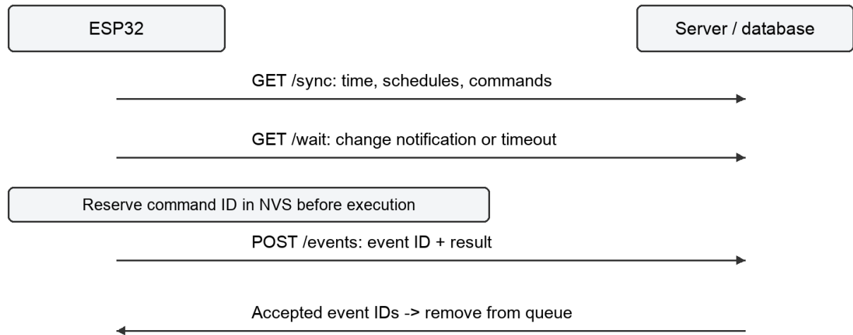
ภาพที่ 3.8 ลำดับการรับข้อมูลและส่งเหตุการณ์ [5], [6]
