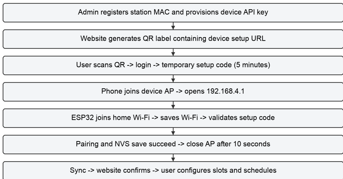
ภาพที่ 3.9 ลำดับตั้งค่าตั้งแต่สร้าง QR จนรับตาราง [5], [6]
