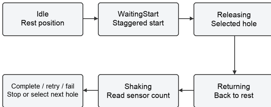
ภาพที่ 3.5 ลำดับสถานะกลไกตาม dispenser_control.cpp [5]
