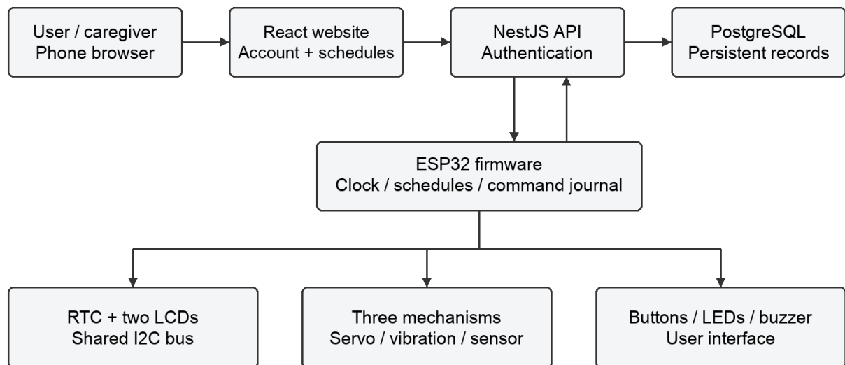
ภาพที่ 3.3 สถาปัตยกรรมระบบตามโค้ดที่ตรวจ [5], [6]
