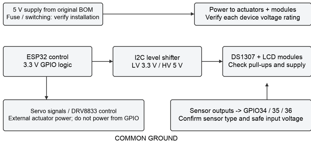
ภาพที่ 3.4 แนวทางจ่ายไฟและแปลงระดับสัญญาณตามข้อมูลที่มี [1]–[3], [5]
