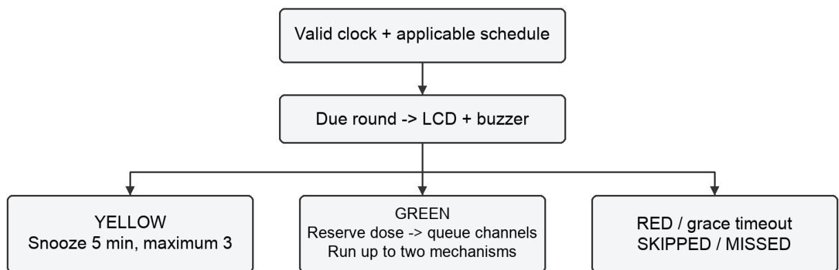
ภาพที่ 3.6 ผังรอบยาและการตอบสนองต่อปุ่ม [5]
