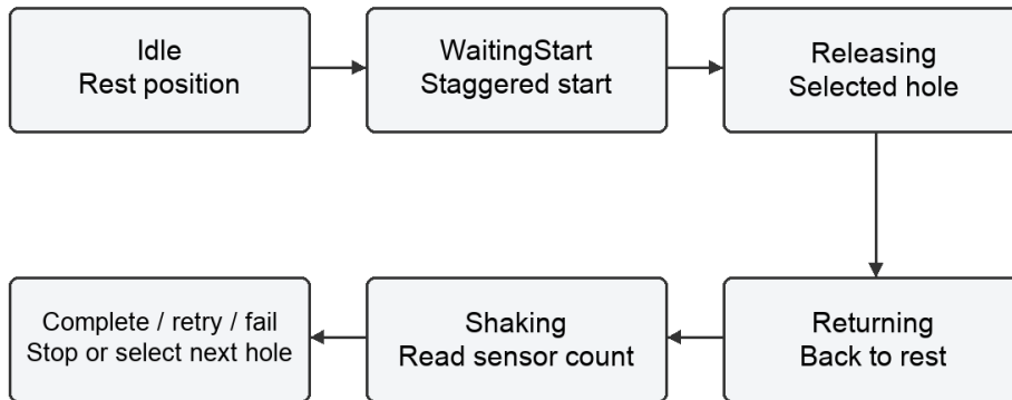
ภาพที่ 3.5 ลำดับสถานะกลไกตาม dispenser_control.cpp [5]
