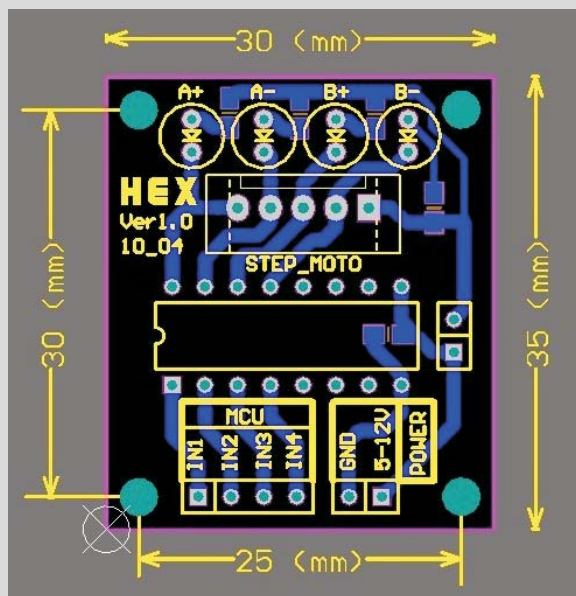
线路板尺寸图
