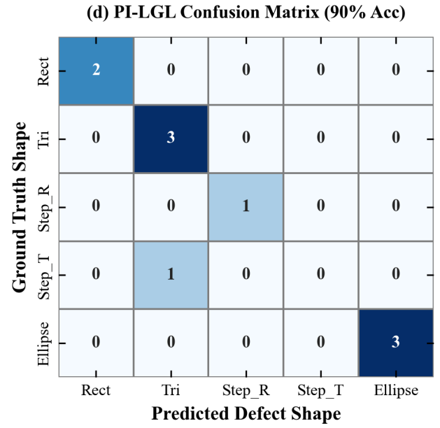
Hình 4 (PI-LGL): Ma trận nhầm lẫn của mô hình PINN đạt độ chính xác 90.0% (đoán đúng 9/10 mẫu kiểm tra mù).
