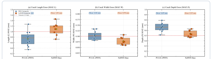
Hình 2 (IEEE Dimension Breakdown): Phân bố Boxplot sai số tuyệt đối MAE của ba chiều không gian Khuyết tật (Bề rộng $W$, Chiều dài $L$, Độ sâu $D$), chứng minh PINN giảm thiểu sai số chiều dài.
