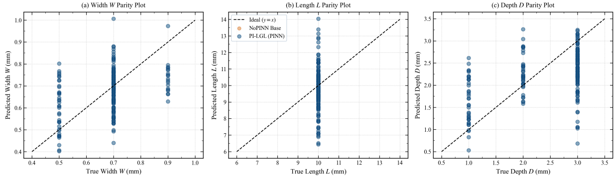
Hình 5 (IEEE Parity Plots - Dự Đoán vs Thực Nghiệm): Biểu đồ đối sánh giá trị dự đoán và giá trị thực đo của Chiều rộng $W$, Chiều dài $L$ và Độ sâu $D$. Hầu hết các điểm mẫu của PINN hội tụ chặt chẽ trong dải biên sai số \pm 0.5 mm dọc theo đường tham chiếu y=x .
