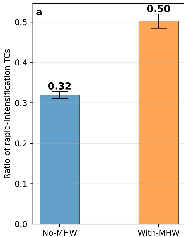
GL: MHW baseline 1982-2011
