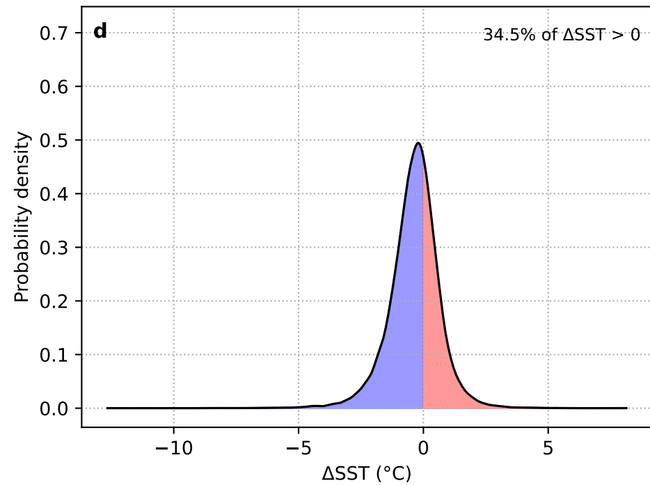
\Delta SST: Day 0 – Day –15 (GL + HYCOM)
