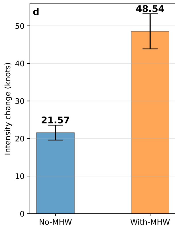
IO: MHW baseline 1982-2011
