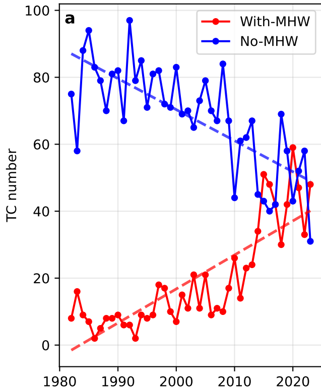
GL: MHW baseline 1982-2011
