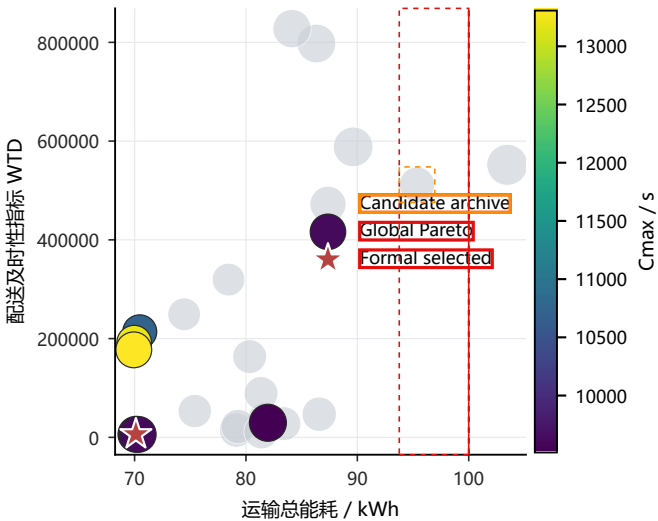
全局候选档案与非支配解
