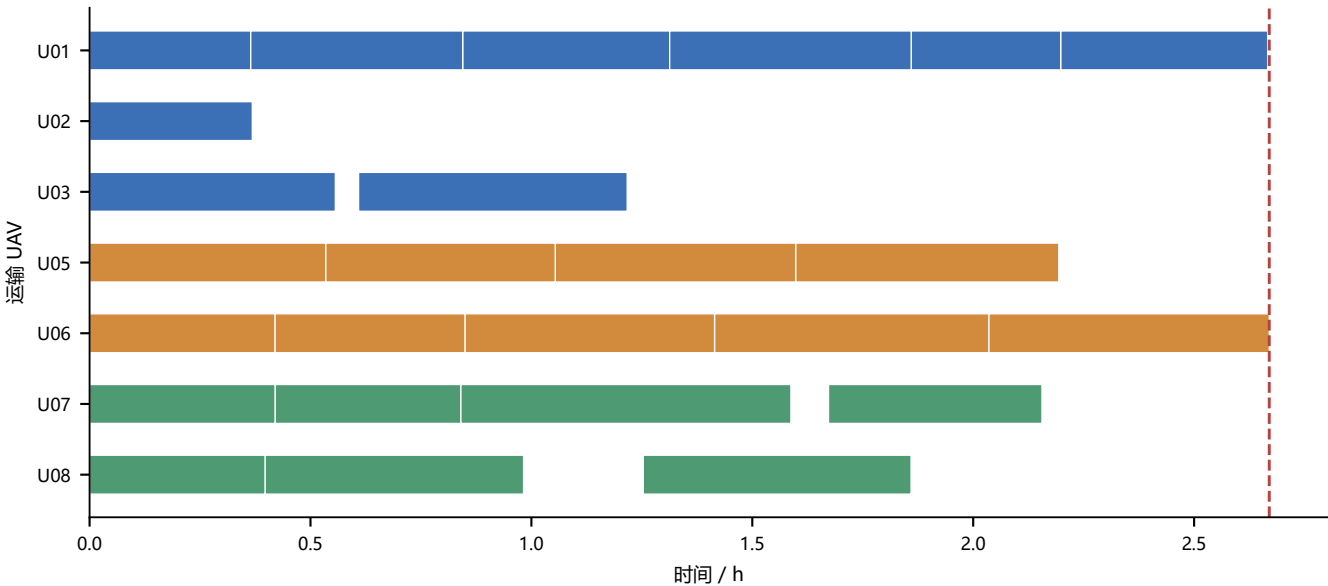
运输 UAV 调度甘特图：并行执行与无重叠占用 蓝 / 橙 / 绿 = A / B / C；红虚线 = C_{max}
