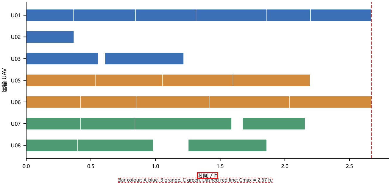
运输 UAV 调度甘特图：并行执行与无重叠占用
