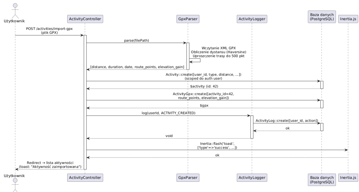
Rysunek 2.4: Diagram sekwencji – import aktywności z pliku GPX
