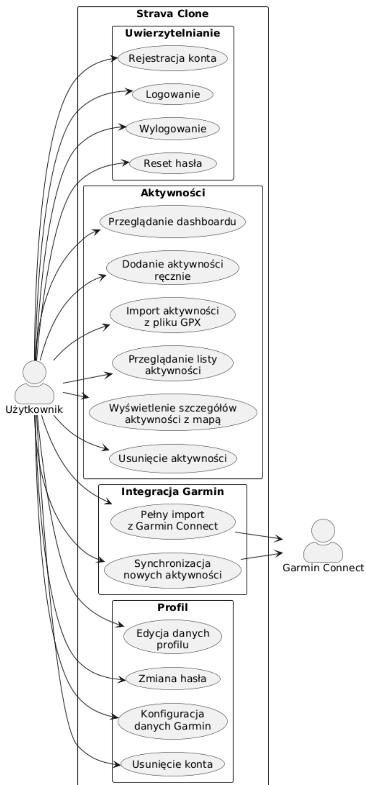
Rysunek 2.1: Diagram przypadków użycia systemu Strava Clone
