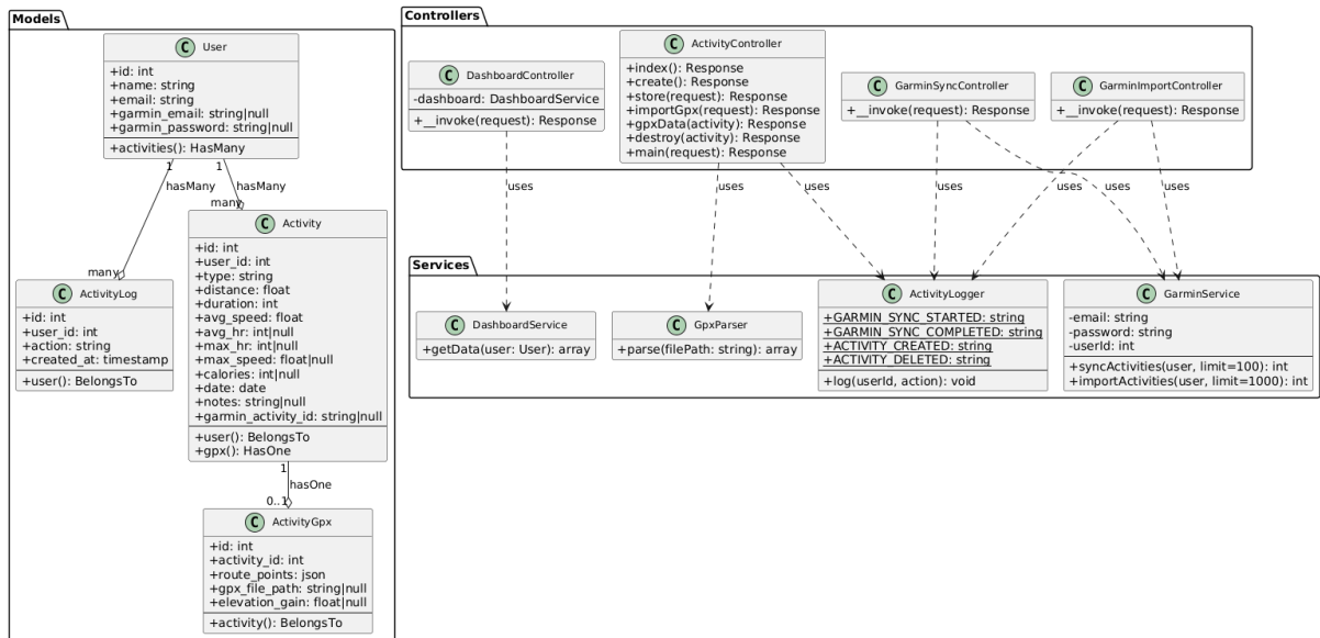
Rysunek 2.3: Diagram klas – modele, serwisy i kontrolery
