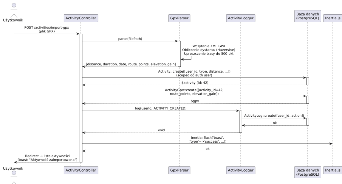
Rysunek 3.4: Diagram sekwencji – import aktywności z pliku GPX
