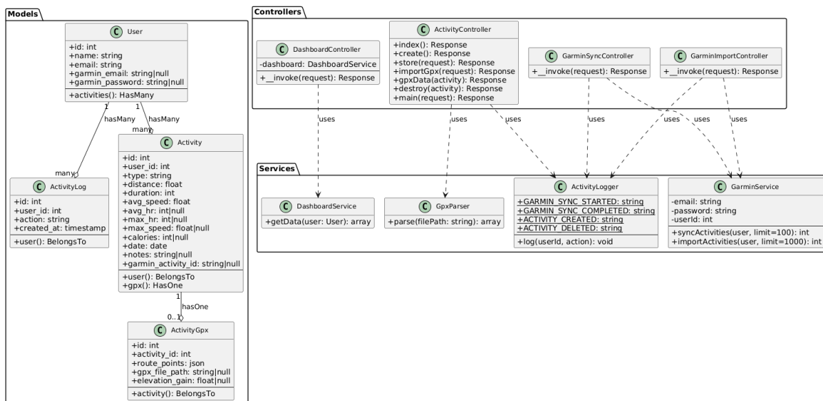
Rysunek 3.3: Diagram klas – modele, serwisy i kontrolery
