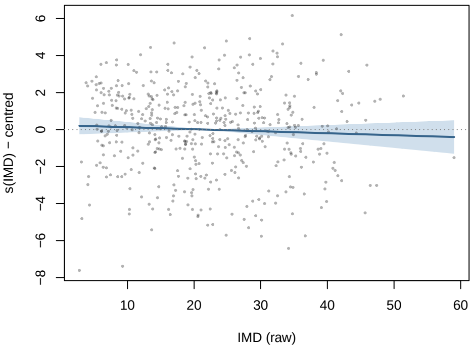
s(IMD) edf=1.0 p=0.37
