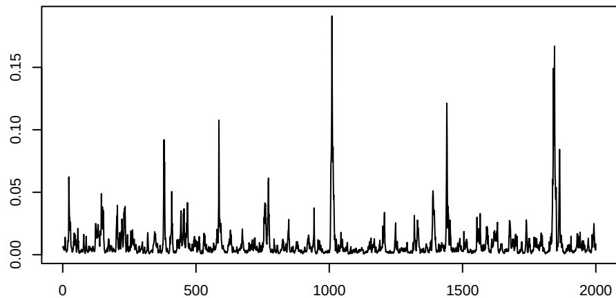
tau2_s[2] (NDVI)
