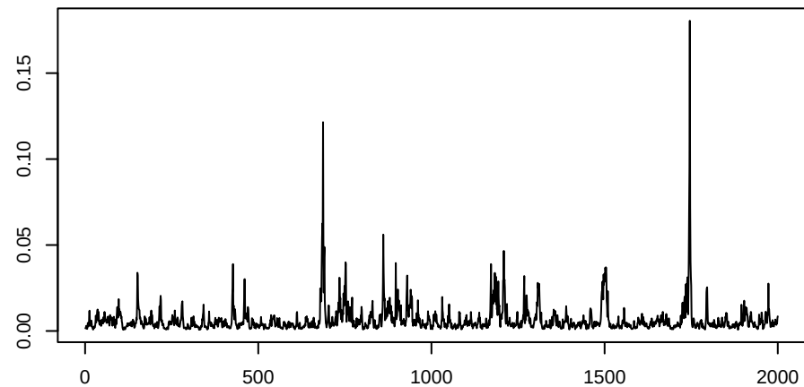
tau2_s[3] (IMD)
