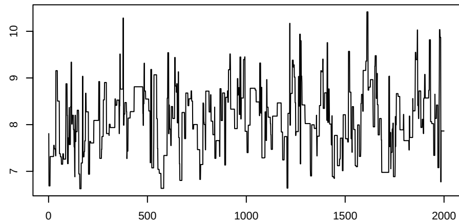
tau2 (spatial)
