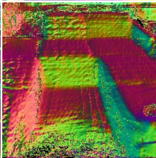
YoNoSplat
