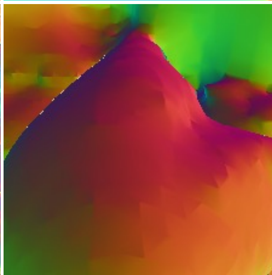
SurfelSplat
