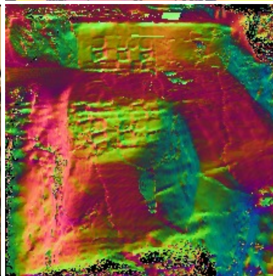
MVSplat
