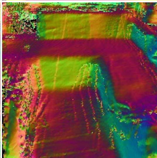
MeshSplat
