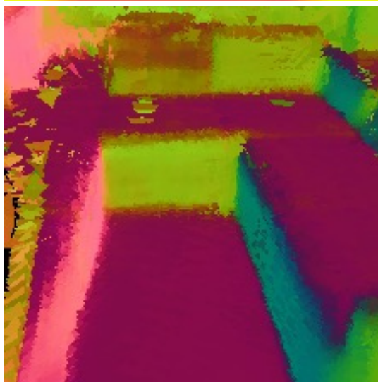
TriSplat
