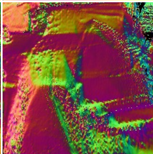
AnySplat
