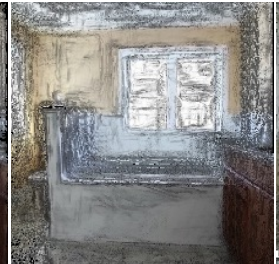
DepthSplat
