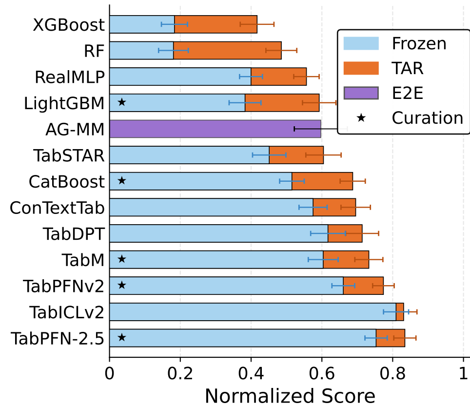
(a) Image-Tabular
