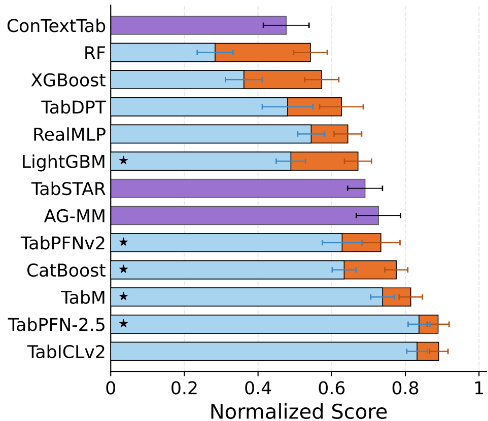
(b) Text-Tabular
