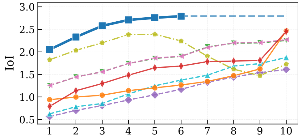
MovieLens-1M — IoI
