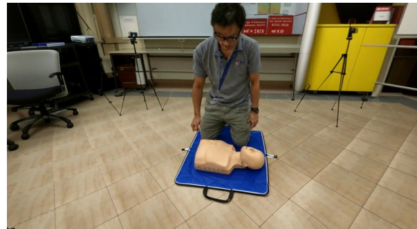
Ours
