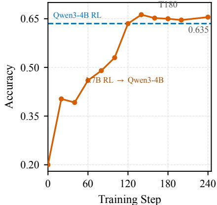
Qwen3 nonthinking: AIME 2025
