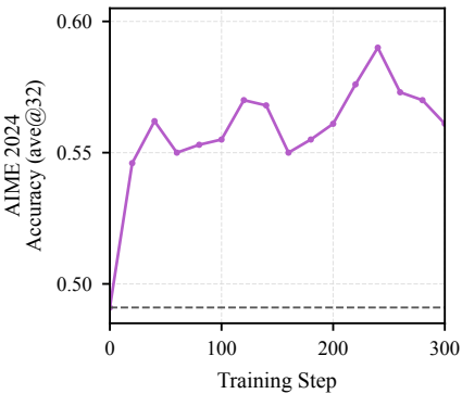
QuestA \rightarrow Qwen3-1.7B
