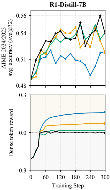
KL 1 KL 1.5 KL 2 Adaptive KL
