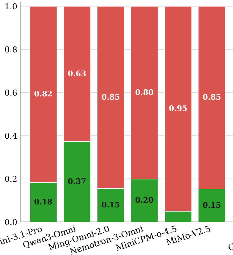
Swap task
