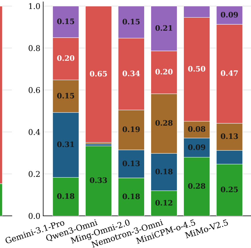
Shift task
